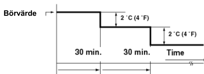
Logik nattsänkning
